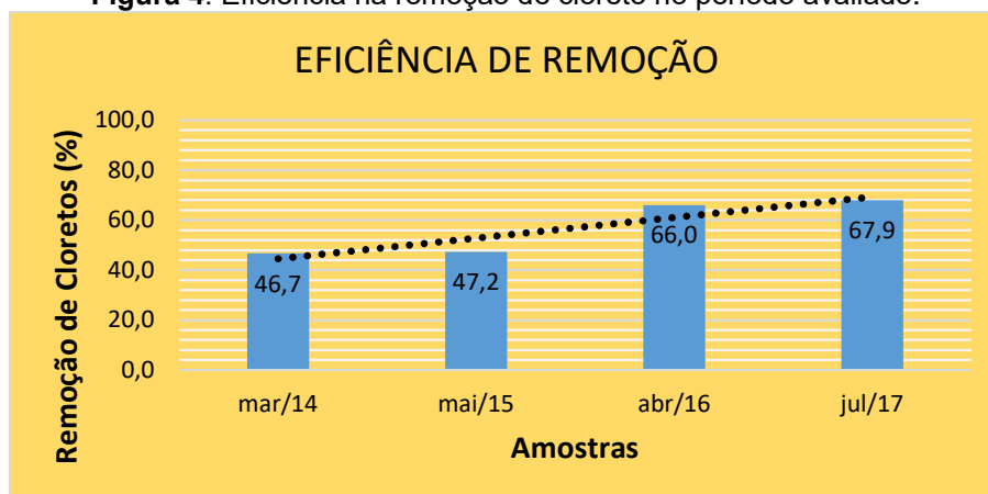
Figura 4. Eficiência na remoção de cloreto no período avaliado.
