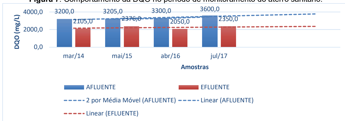
Figura 7. Comportamento da DQO no período de monitoramento do aterro sanitário.
